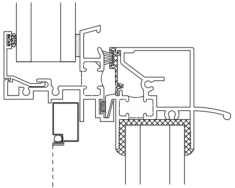
② INTERLOCK
